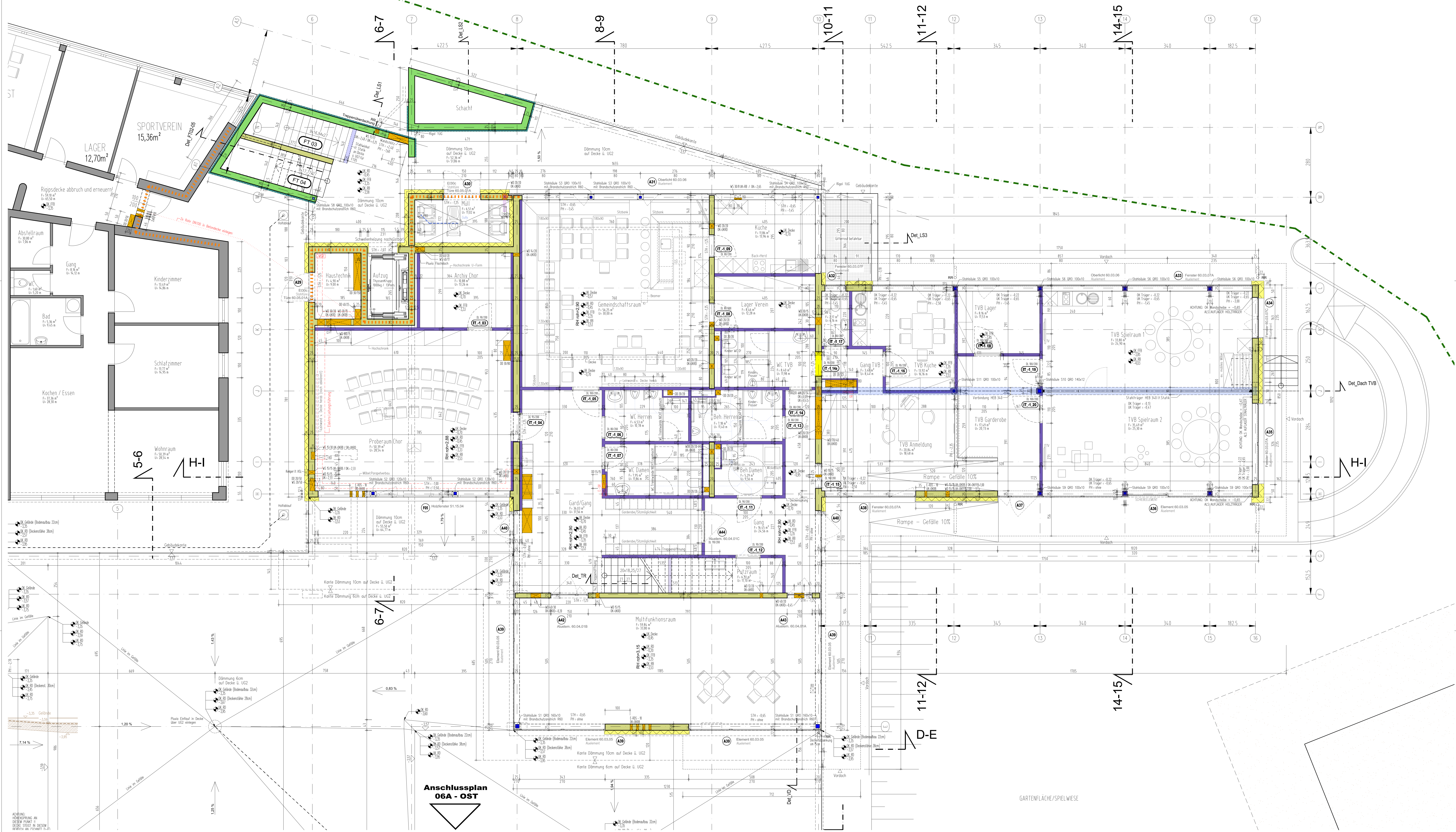
GRUNDRISS UG1
